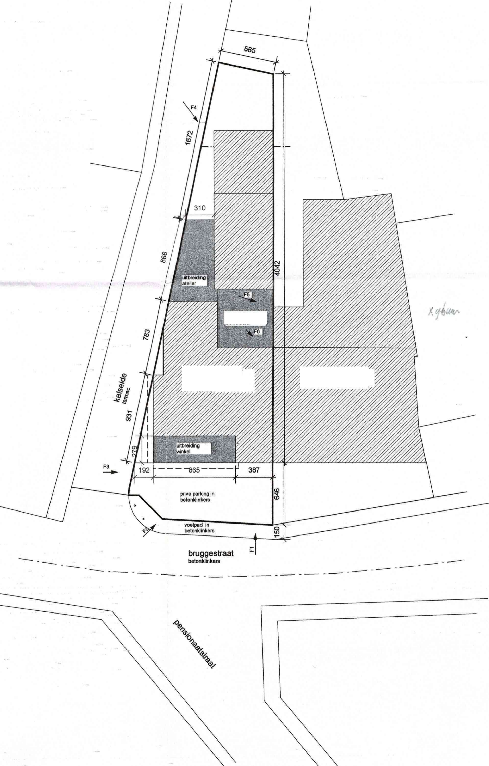
VERKAVELINGSPLAN ONTWORPEN TOESTAND 1/200
